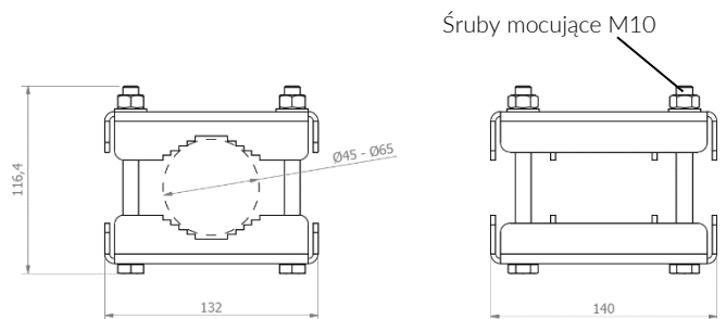
US0 SUMO/SOLARIS uchwyt do montażu na słupie
